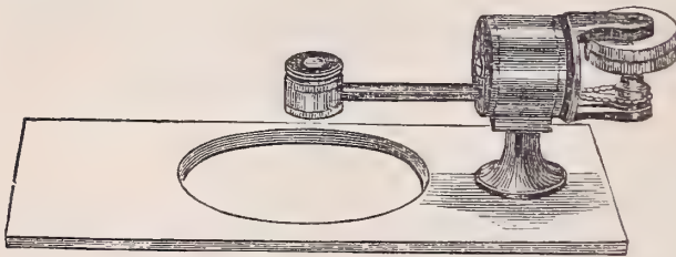
FIG. 246.—Beck's disc-holder.
