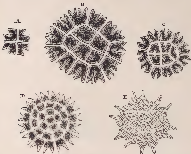
FIG. 380.—Various species (?) of Pediastrum : A, P. tetras ; B, C, P. Ehrenbergii ; D, P. pertusum ; E, empty frond of P. granulatum .
